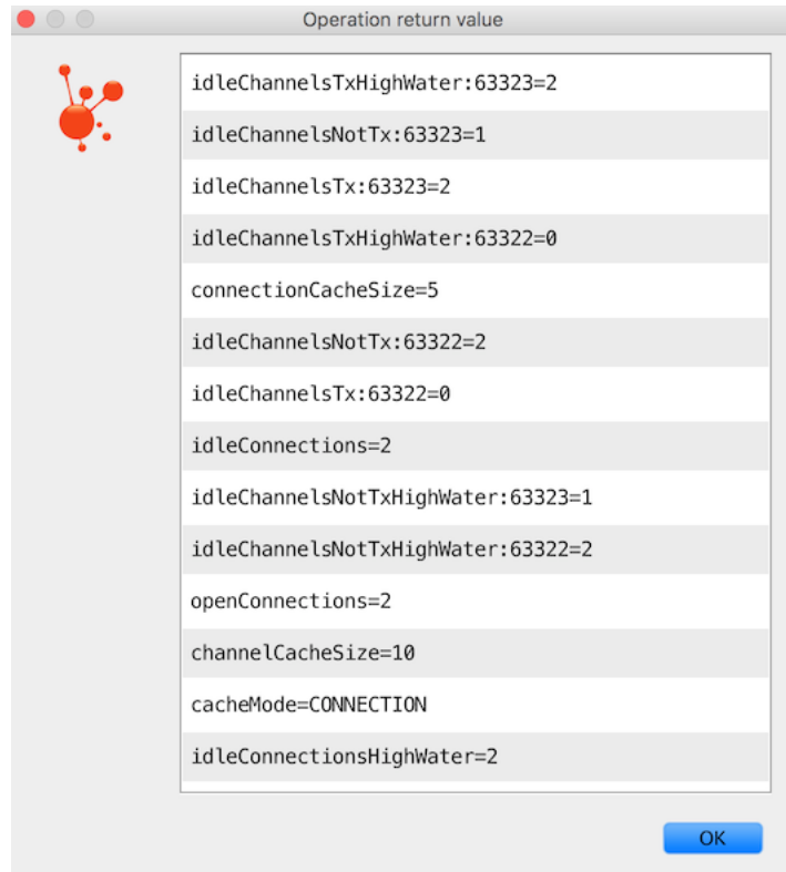
Figure 3.1. JVisualVM Example
