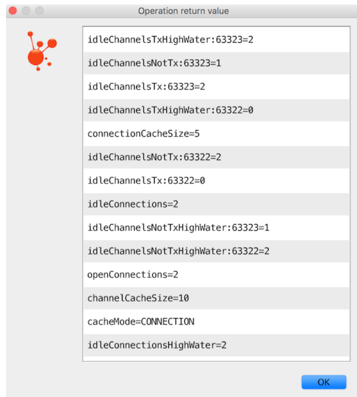
Figure 3.1. JVisualVM Example
